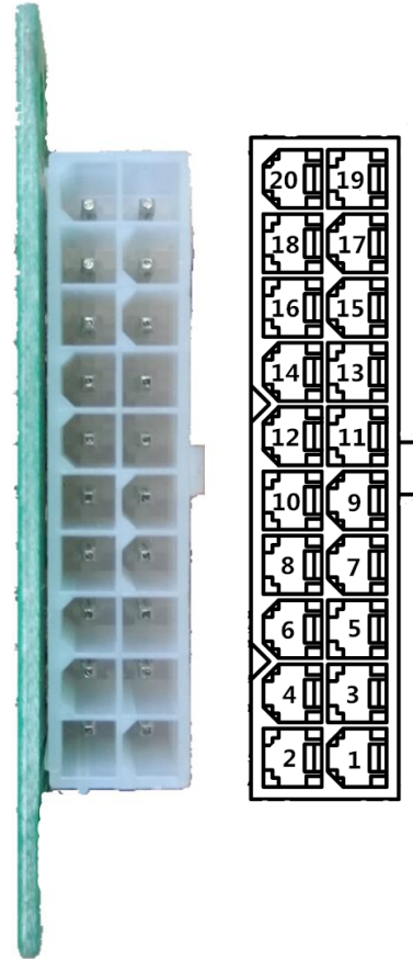
图 2.5 J5 端子序号图
