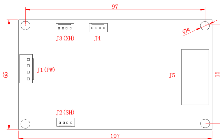
图 2.3 BL2000-HXJ-V9(1)尺寸图（单位 mm）
