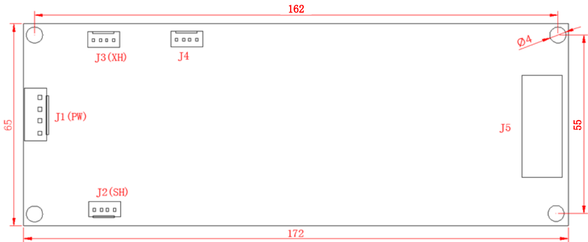
图 2.6 BL2000-HXK-V9(1) 尺寸图 (单位 mm)
